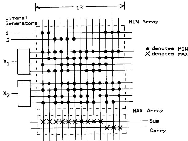
Fig. 4. Adder using Type 1 PLA.
