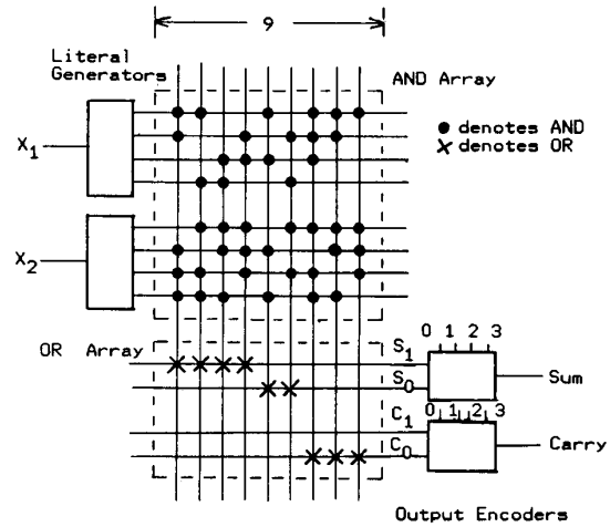
Fig. 8. Adder using Type 2 PLA.
